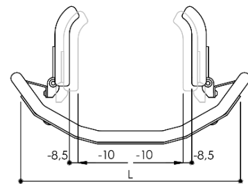
Interne laterale steun aan rugleuning, breedte aanpasbaar (-8,5 ÷ -10cm)
