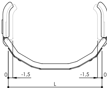
Interne laterale steun aan rugleuning, breedte aanpasbaar (0 ÷ -1,5cm)
