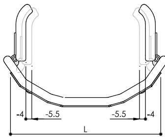
Interne laterale steun aan rugleuning, breedte aanpasbaar (-4 ÷ -5,5cm)
